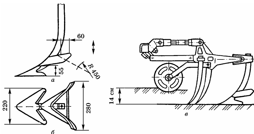
Рис. 23. Схематичне зображення робочих органів швидкісного підгортача: а — лапа; б — секція; в — загальна схема
