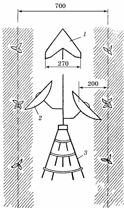
Рис. 22. Схема розміщення робочих органів в агрегаті для післясходового обробітку у міжряддях і захисних смугах на посівах кукурудзи, сояшнику: 1 — стрілочаста лапа; 2 — дисковий загортач-підгортач; 3 — полільна борінка
