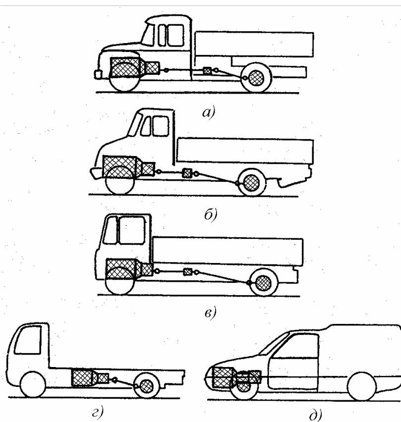
Рис. 1.9. Компоновочные схемы грузовых автомобилей общего назначения: a - капотная; б - полукапотная; в - бескапотная (кабина над двигателем); г - с двигателем внутри колесной базы; д - на основе конструкции легкового автомобиля
