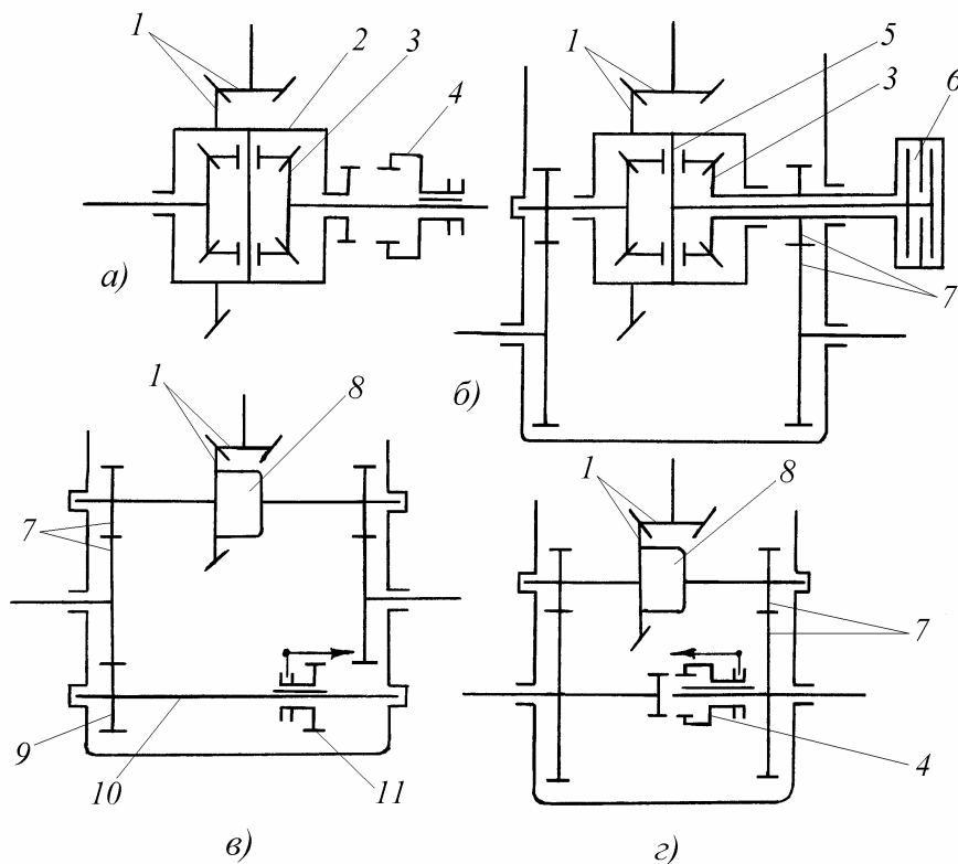
Рис. 6.6. Способы блокировки межколесного дифференциала:
