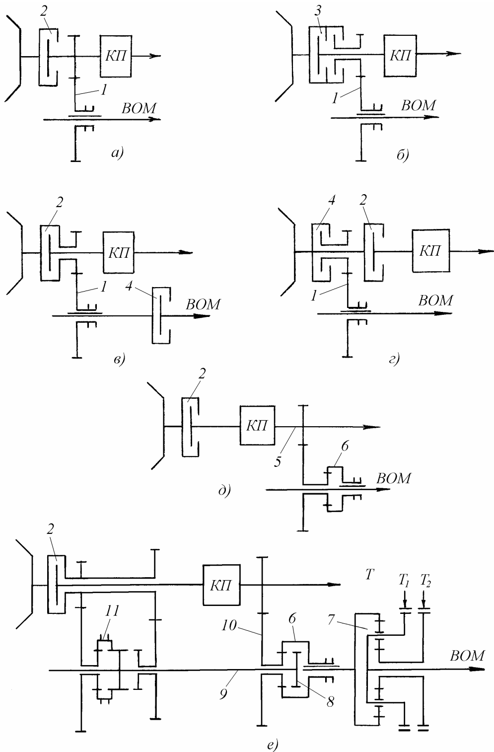
Рис. 12.14. Схемы приводов ВОМ:
