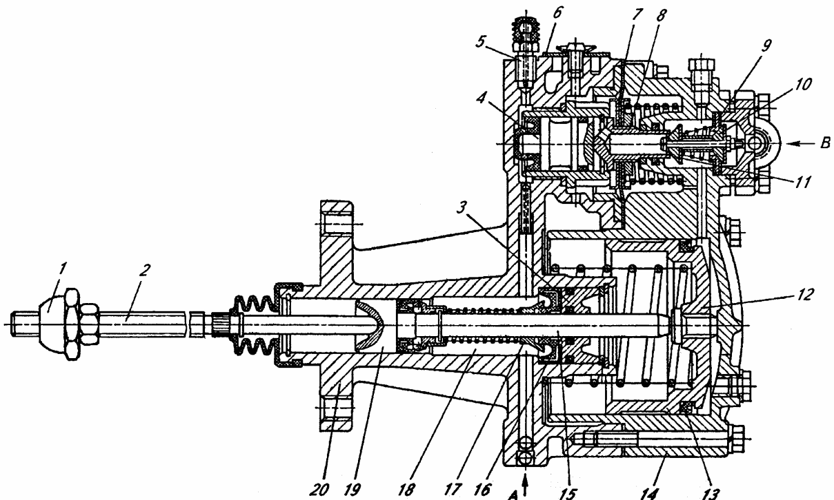
Рис. 3.14. Пневматический усилитель:
