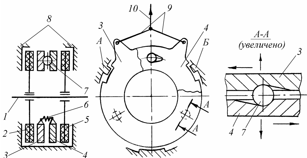
Рис. 11.4. Схема закрытого дискового тормоза с сервоусилением:
