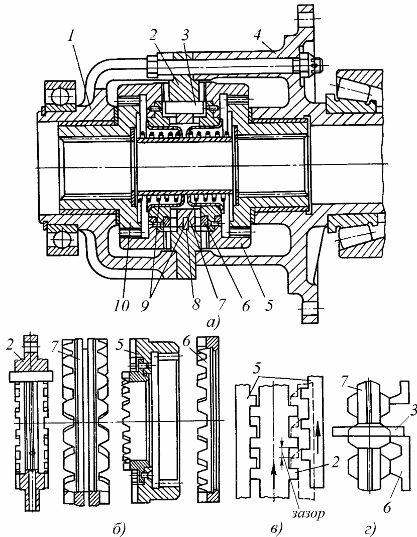
Рис. 6.9. Механизм распределения мощности с муфтами свободного хода:
