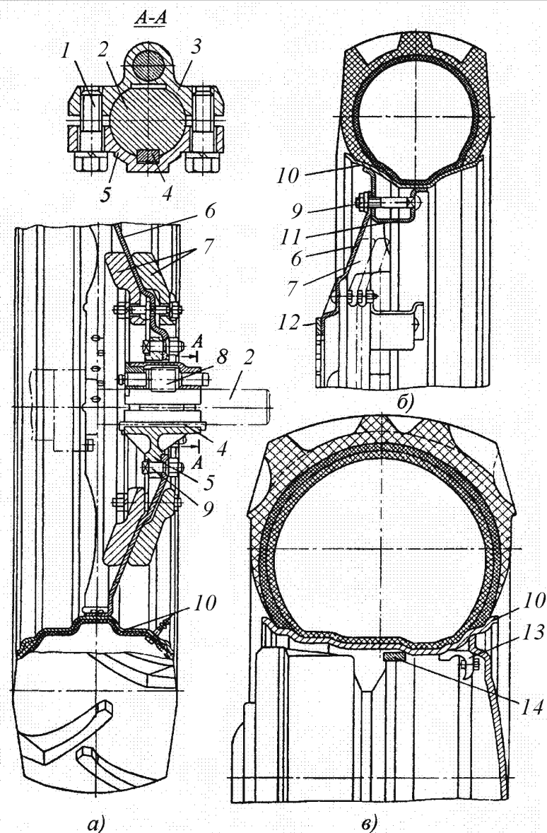
Рис. 8.5. Ведущие колеса тракторов:
