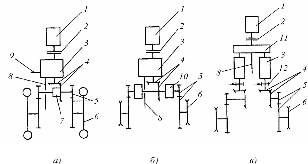
Рис. 2.1. Принципиальные структурные кинематические схемы ступенчатых трансмиссий тракторов:
