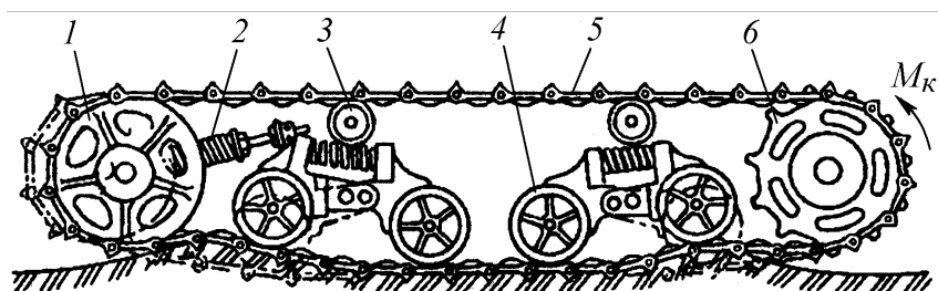
Рис. 8.11. Гусеничный движитель:
