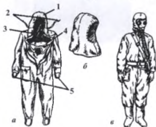
Іл. 37.5. Захисний фільтрувальний одяг (ЗФО-58): а — комбінезон: 1 — капюшон; 2 — шнурки для затягування капюшона; 3 — головний клапан; 4 — нагрудний клапан; 5 — штрипки підрукавників; б — підшоломник; в — одягнений ЗФО-58
