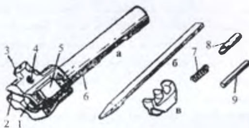
Іл. 13.4. Затвор: а — корпус затвора; б — ударник; в — викидач 1 — чашечка для дна гільзи; 2 — виріз для викидача; 3 — спрямовуючий виступ; 4 — отвір для осі викидача; 5 — бойовий виступ; 6 — поздовжній паз; 7 — пружина викидача; 8 — вісь викидача; 9 — штифт ударника
