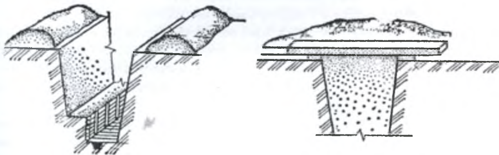
Іл. 35.1. Відкрита та перекрита щілини
