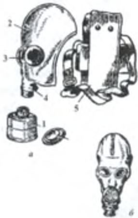
Іл. 36.6. Протигаз ЦП-5
