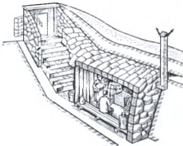
Іл. 35.2. Погріб, пристосований під ПРУ
