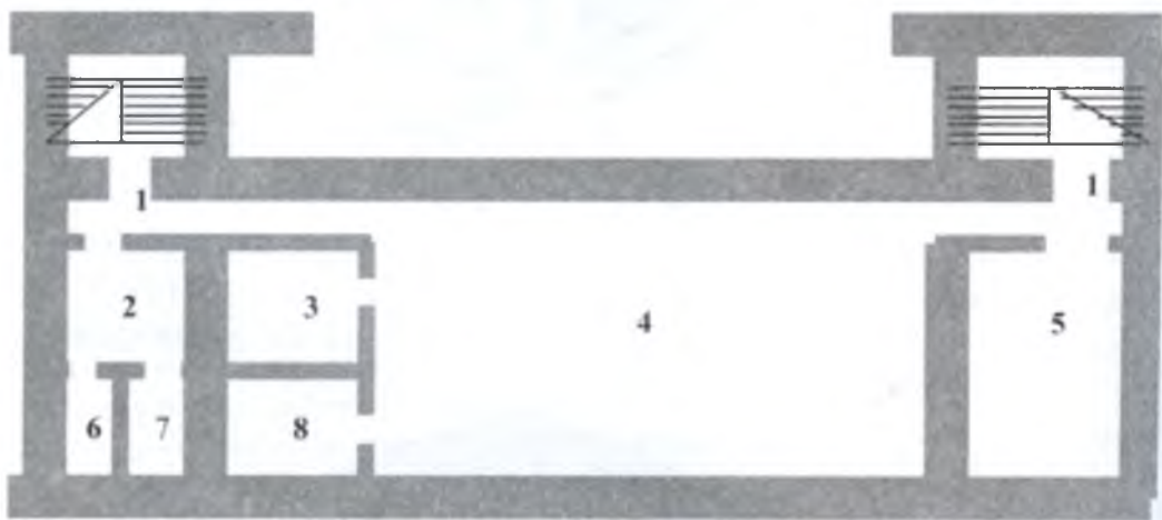
Іл. 35.4. Схема протирадіаційного укриття (варіант)
