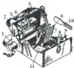
Іл. 34.10. Військовий прилад хімічної розвідки (ВПХР): 1 — ручний насос; 2 — плечовий ремінь з тасьмою; 3 — насадка до насоса; 4 — захисні ковпачки для насадки; 5 — протидимні фільтри; 6 — патрон грілки; 7 — електричний ліхтар; 8 — корпус грілки; 9 — штир; 10 — лопатка; 11 — індикаторні трубки в касетах
