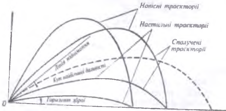
Іл. 11.4. Траєкторії польоту кулі
