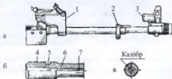
Іл. 13.1. Ствол автомата: а — зовнішній вид ствола автомата; б — казенна частина в розрізі; в — розріз ствола; 1 — колодка прицілу; 2 — кільце цівки; 3 — колодка мушки; 4 — патронник; 5 — виїмка для штифта ствола; 6 — кульовий вхід; 7 — нарізна частина
