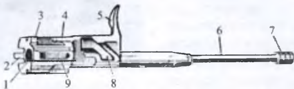
Іл. 13.3. Затворна рама зі штоком: 1 — канал для затвора; 2 — запобіжний виступ; 3 — виступ для опускання важеля автоспуску; 4 — паз для відгинів ствольної коробки; 5 — рукоятка; 6 — шток; 7 — газовий поршень; 8 — фігурний виріз; 9 — паз для виступу відбивача
