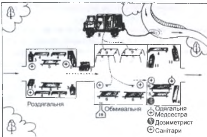
Іл. 39.3. Санітарно-обмивальний пункт на базі ДДА-66: 1 — засоби для надання невідкладної медичної допомоги; 2 — засоби для дегазації; 3 — мішки для зараженого одягу; 4 — лавки для легкопоранених; 5 — ноші санітарні; 6 — ноші сітчасті для обробки тяжкопоранених; 7 — ящик для протигазів, знятих при переході в обмивальню; 8 — дезінфекційно-душова установка на автомобілі (ДДА-66); 9 — душові пристрої для легкопоранених; 10 — поглинальний колодязь; 11 — чиста білизна й одяг
