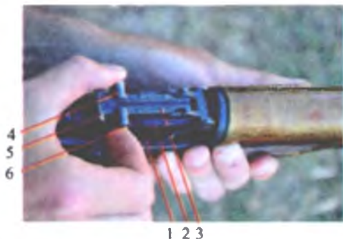
Іл. 13.2. Приціл автомата: 1 — колодка прицілу; 2 — сектор; 3 — прицільна планка; 4 — хомутик; 5 — гривка прицільної планки; 6 — засувка хомутика
