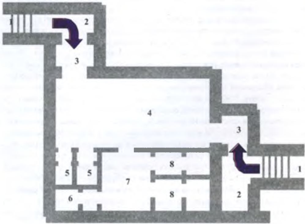
Іл. 35.5. План-схема окремо розташованого сховища:
