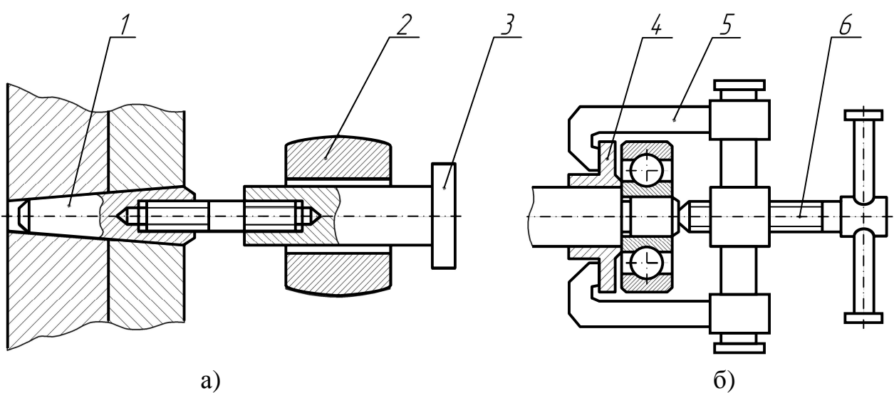
Рис. 11.6. Знімачі: а – для демонтажу штифтів з різьбою; б – для демонтажу підшипників, кілець, втулок; 1 – штифт; 2 – вантаж; 3 – упор; 4 – деталь, розташована за підшипником (втулка); 5 – затискач; 6 – гвинт
