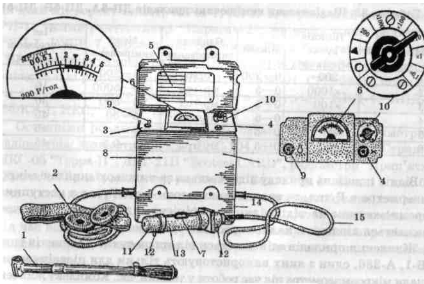
Рис. 11. Прилад ДП-5В:
