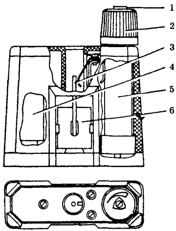
Рис. 15. Зарядний пристрій ЗД-6 до комплексу ІД-1: 1 — тригранник; 2 — ручка; 3 — зарядно-контактне гніздо; 4 — розрядник; 5 — перетворювач; 6 — джерело
