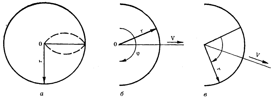
Рис. 31. Нанесення зон зараження СДЯР на карту (схему): а — при швидкості вітру < 1 м/с; б — при швидкості вітру 1 м/с; в — при швидкості вітру > 1 м/с
