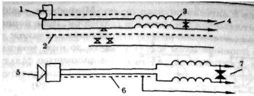
Рис. 89. Схема захисту ліній мікрофонів і репродукторів: 1 — мікрофон; 2 — екранована пара проводів; 3 — швидкодіючий варистор; 4 — до радіоустановки; 5 — зовнішній репродуктор; 6 — екранована пара проводів; 7 — до радіоустановки
