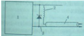
Рис. 87. Типовий захист обладнання з Живленням постійним током: — джерело постійною струму; 2 — адіочастотна дросельна катушка; 3 — швидкодіючий варистор; 4 — екранований провід
