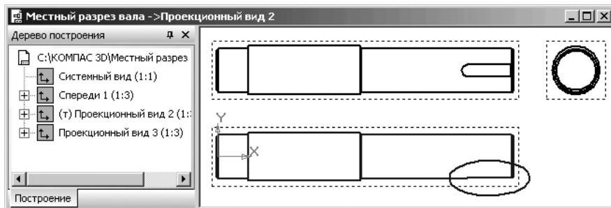
Рис. 4.145. Построение замкнутого контура в виде эллипса для местного разреза на текущем виде Проекционный вид 2
