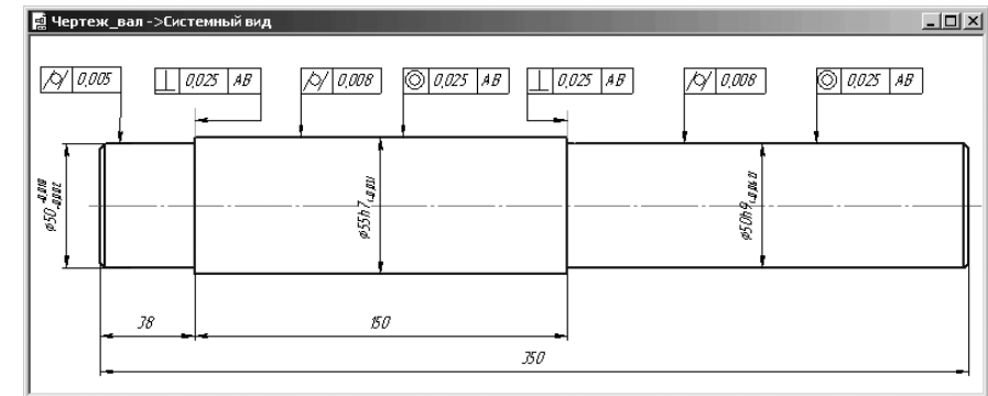
Рис. 4.113. Знаки обозначения допусков форм поверхности для вала
