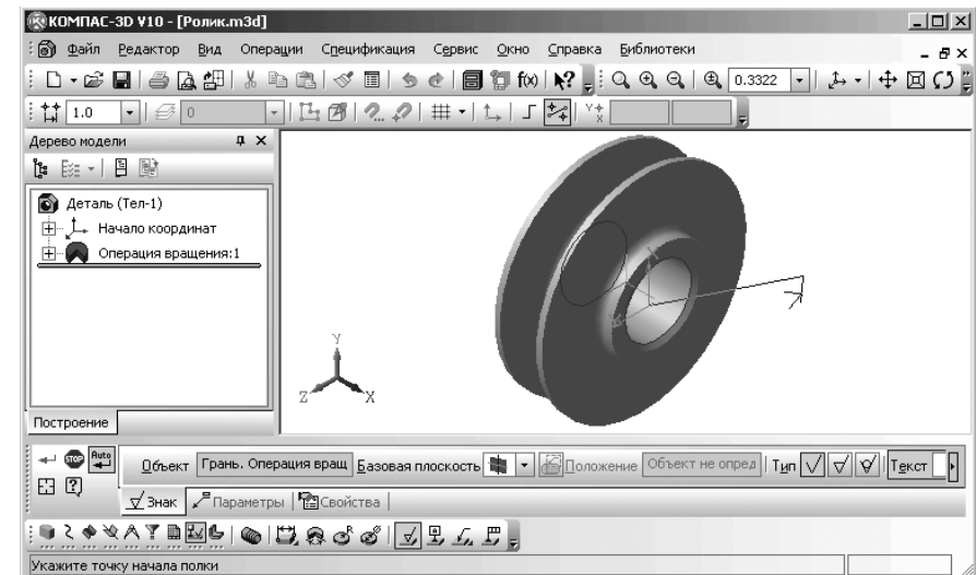
Рис. 3.143. Главное окно системы в режиме завершения простановки диаметрального размера отверстия ролика
