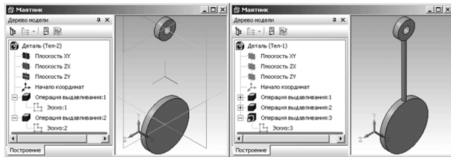
Рис. П1.5. Пример проектирования детали (маятника) с нескольких сторон
