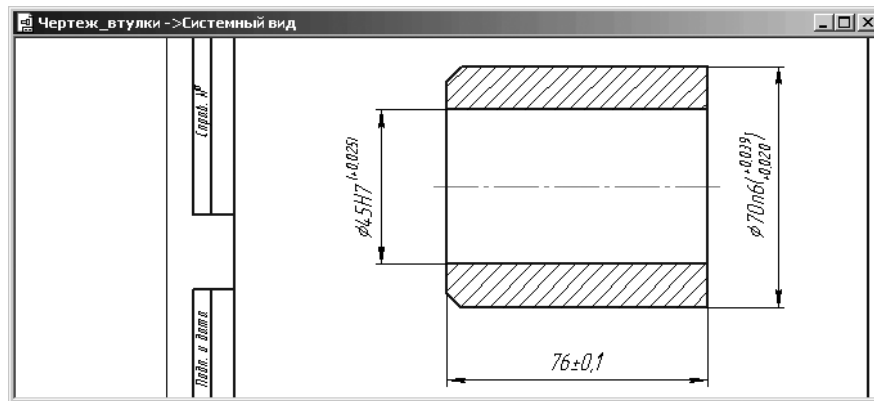
Рис. 4.81. Втулка с установленными размерами
