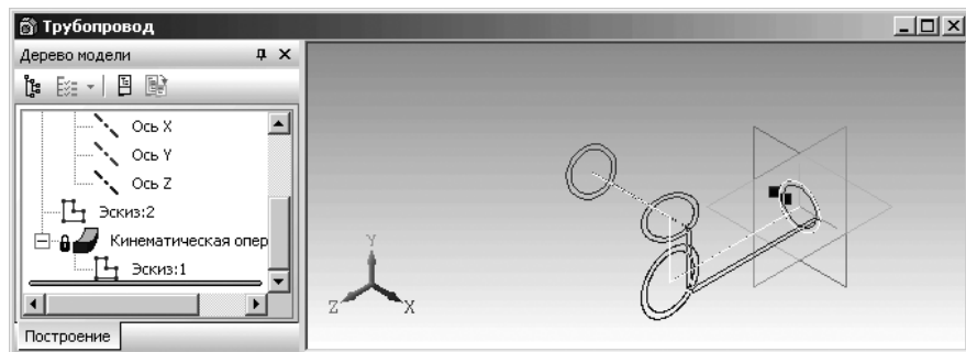
Рис. 2.125. Фантом трубопровода с установленной толщиной стенки
