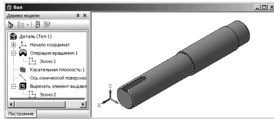
Рис. 4.135. Модель трехступенчатого вала
