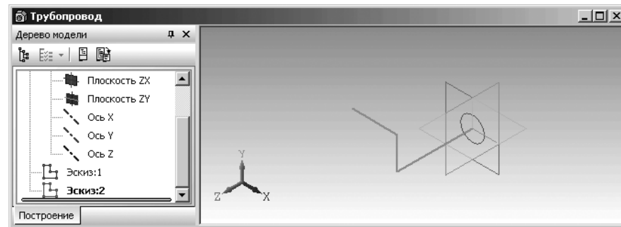
Рис. 2.120. Окно модели Трубопровод после создания эскиза сечения Эскиз:1 и эскиза траектории Эскиз:2
