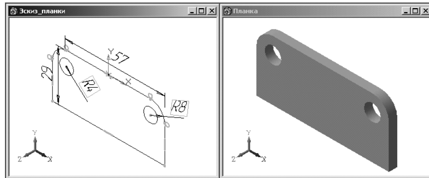
Рис. 1.52. Пример эскиза планки и модель планки после выдавливания
