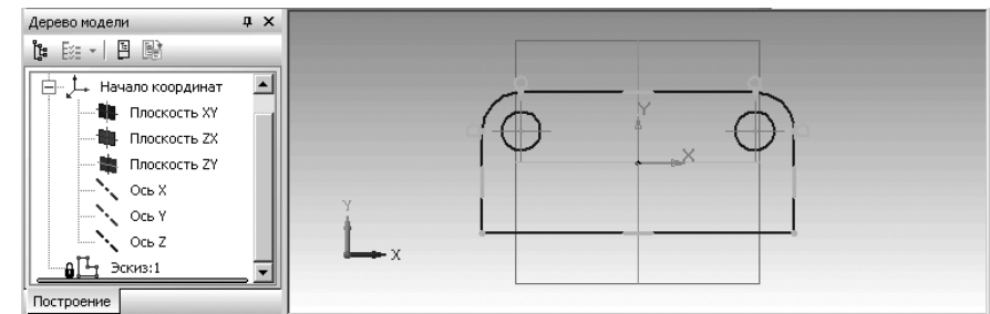
Рис. 2.82. Эскиз стопорной планки
