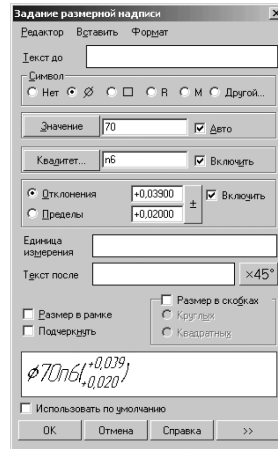
Рис. 4.80. Установка внешнего диаметра Втулки
