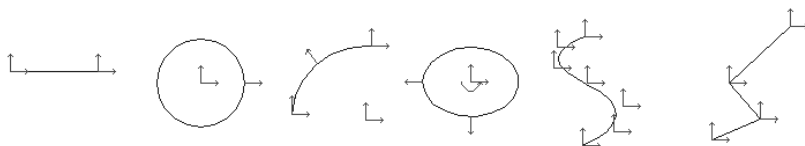
Рис. 1.98. Значки, отражающие степени свободы для наиболее распространенных объектов: отрезка, окружности, дуги, эллипса, NURBS кривой, ломаной кривой
