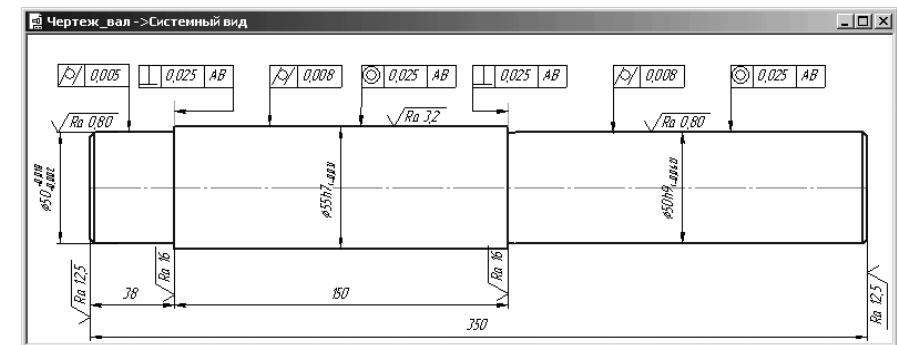
Рис. 4.116. Вал с знаками обозначения шероховатости и допуска формы
