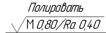
Рис. 5.7. Структура обозначения шероховатости с изменением № 3, 2003
