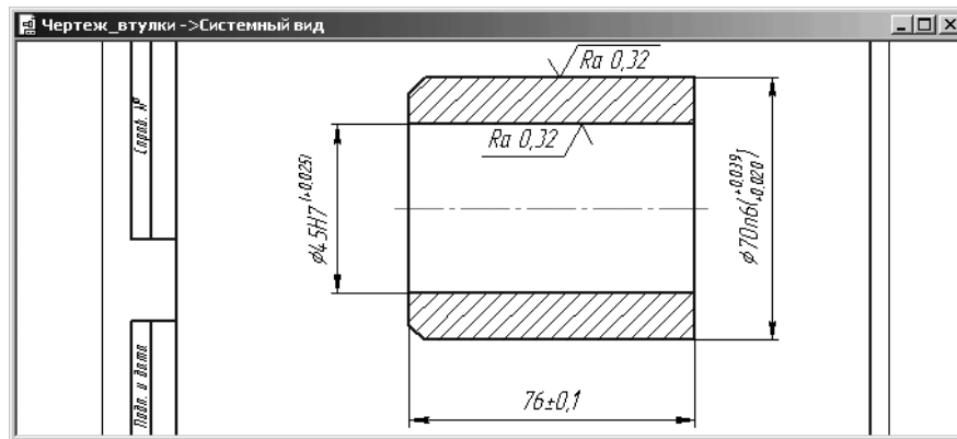
Рис. 4.85. Втулка после простановки шероховатости
