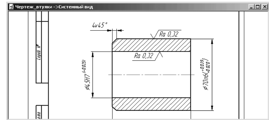
Рис. 4.87. Втулка с установленными размерами и значениями шероховатости
