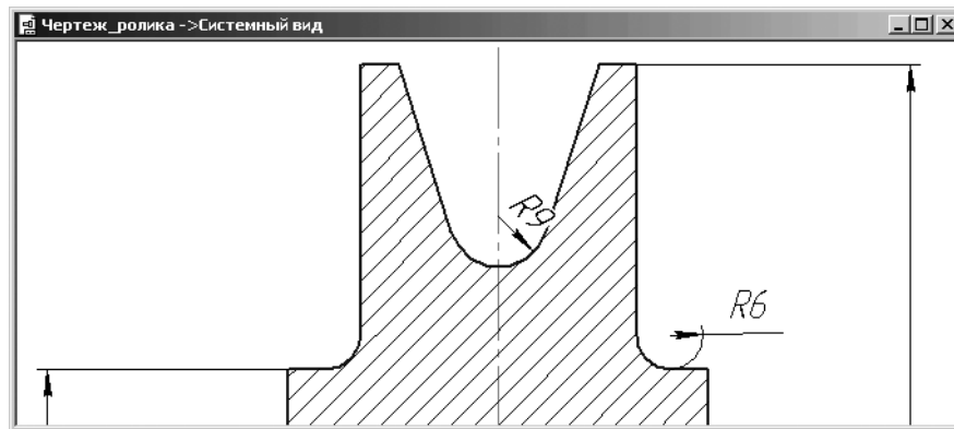
Рис. 4.54. Результаты простановки радиальных размеров канавки ролика и скругления на бобышке в окне чертежа
