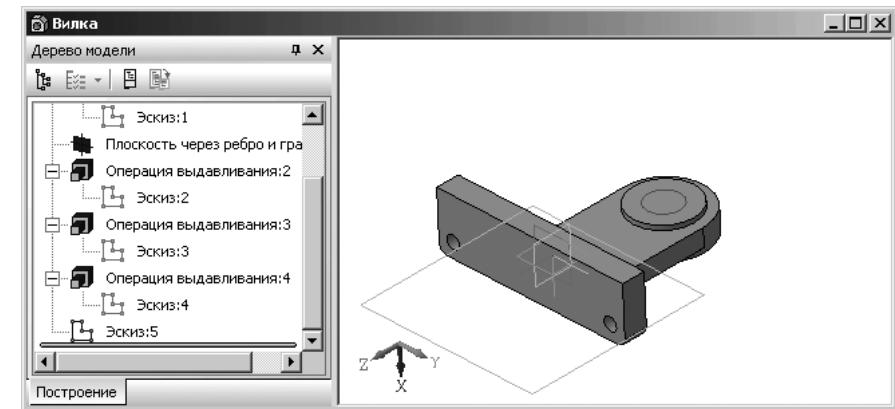
Рис. 3.69. Результат построения эскиза отверстия на бобышке
