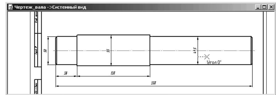
Рис. 4.104. Установка линейных размеров на валу
