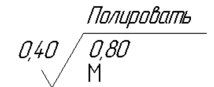
Рис. 5.6. Структура обозначения шероховатости до изменения № 3, 2003
