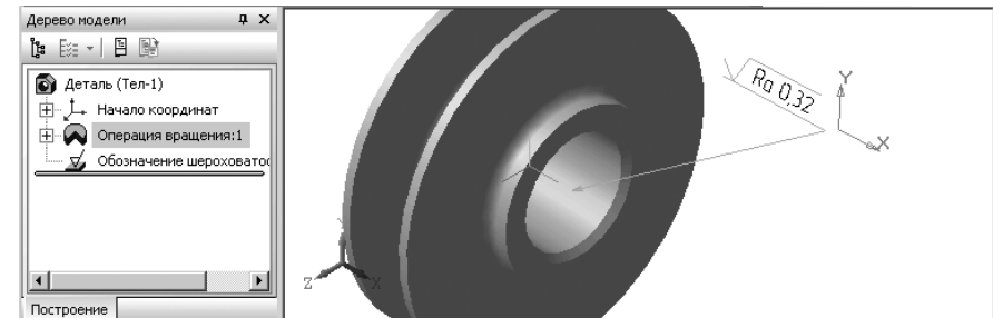
Рис. 3.146. Результат простановка значения шероховатости грани ролика нажмите на клавишу Esc для завершения простановки шероховатости
