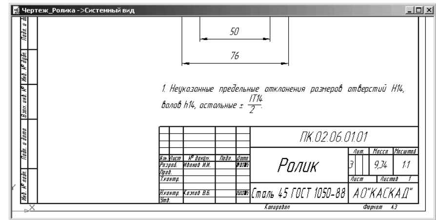
Рис. 5.83. Перенос уменьшенной страницы Технические требования на чертеж
