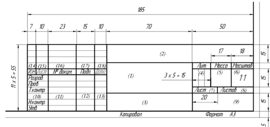
Рис. 5.32. Форма, размеры и содержание граф основной надписи согласно ГОСТ 2.104
