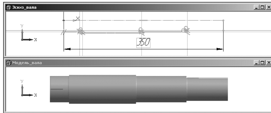
Рис. 1.51. Пример эскиза вращения для построения детали и сама деталь, показанная Спереди
