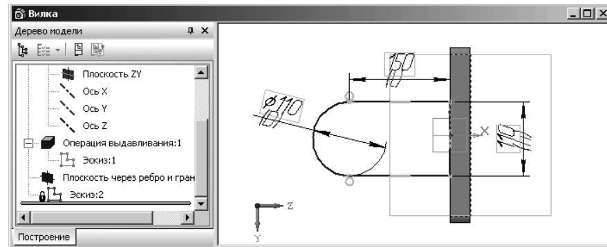
Рис. 3.59. Результат параметризации размеров эскиза проушины
