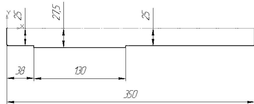
Рис. 2.37. Эскиз вращения для создания модели вала
