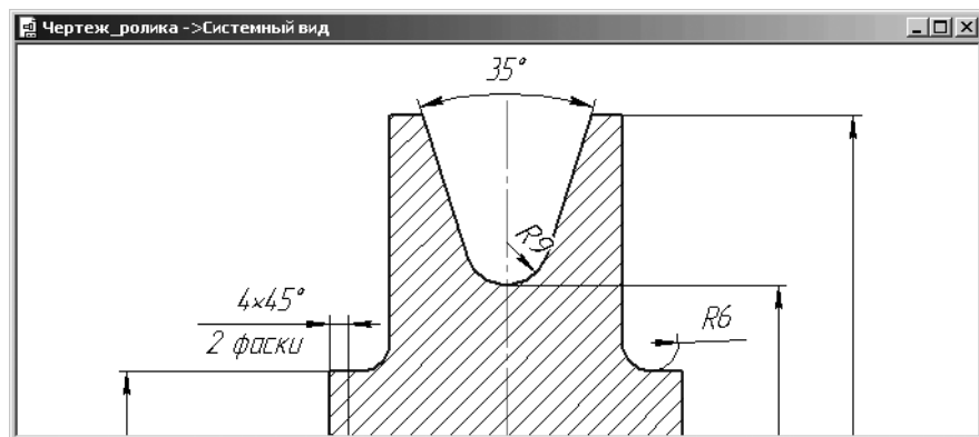
Рис. 4.61. Результат простановки текста под размерной надписью фаски
