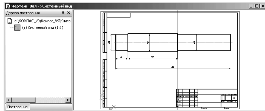
Рис. 4.121. Вал с линейными размерами на форматке А3 с горизонтальной ориентацией в масштабе 1:1
