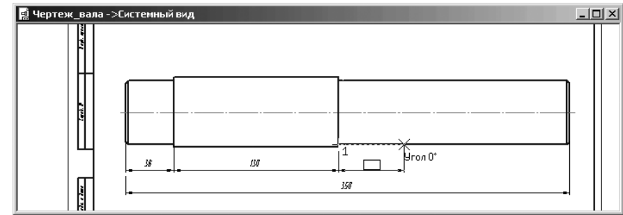
Рис. 4.103. Представление размеров общей длины вала и его ступеней
