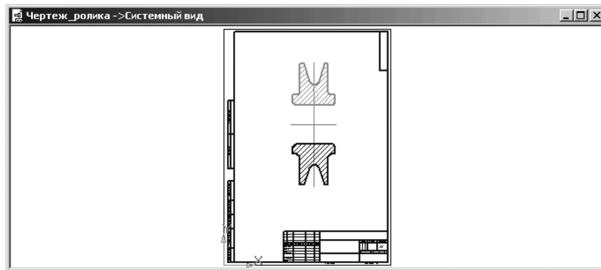
Рис. 4.43. Симметричное отображение верхней половины ролика
